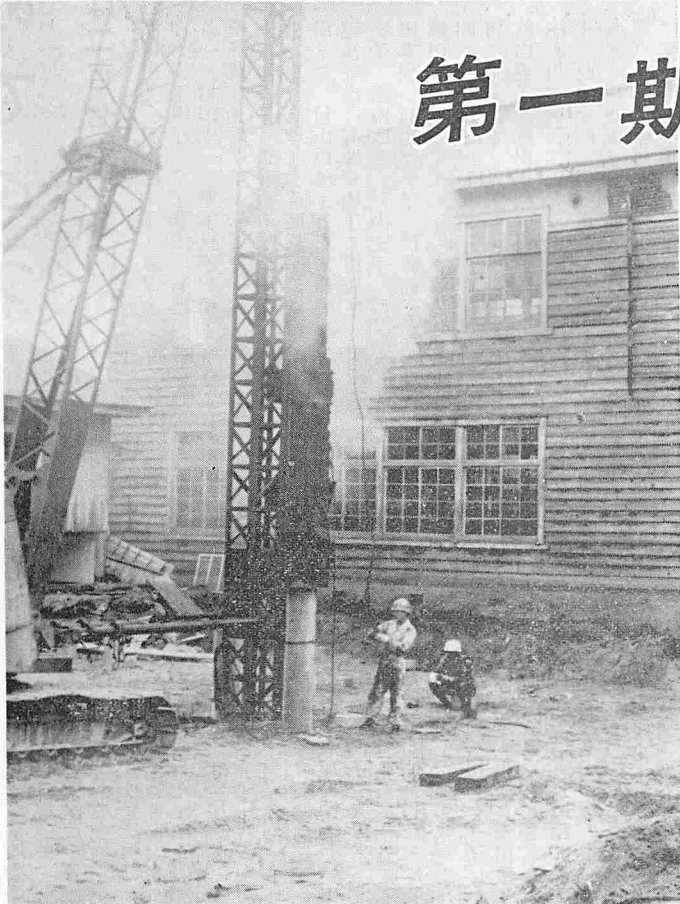
▲基礎クイ打ちをしている工事現場
