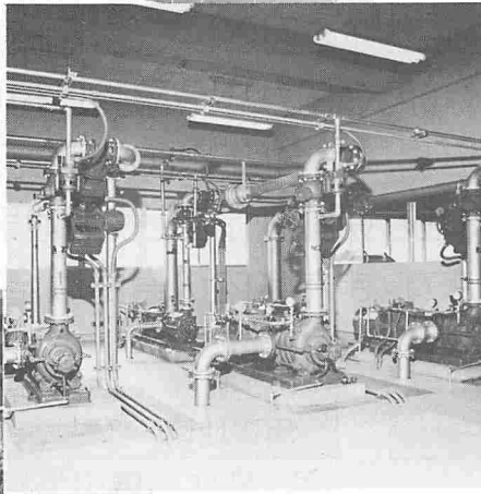
◁ 除鉄 除マンガン装置
